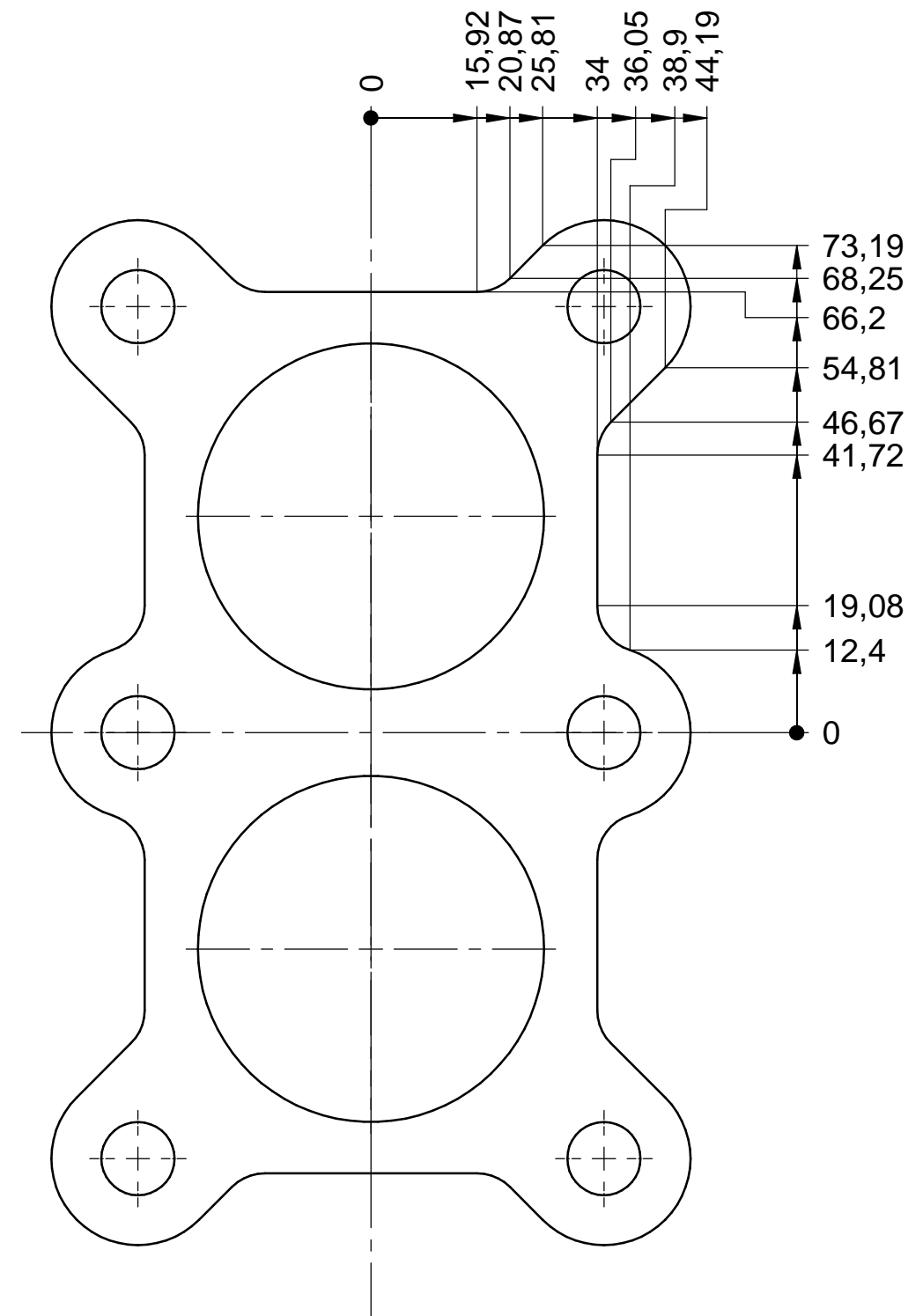
AGG-Auspuffflansch
